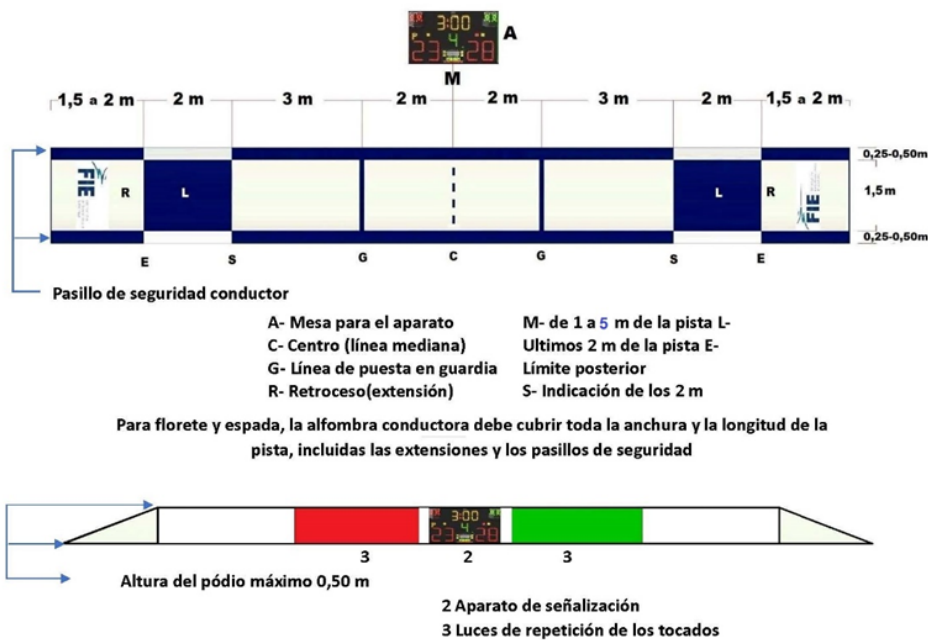
Figura 1 - PISTA PARA LAS FINALES (altura de la pista máximo 0,50 m)
